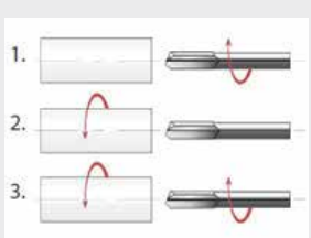
Tool and workpiece rotation Werkzeug- und Werkstückrotation
